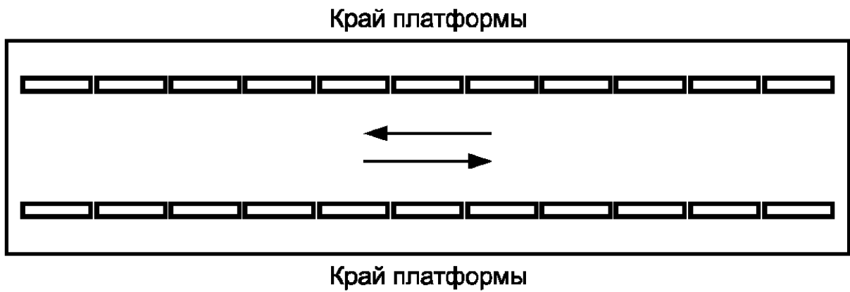
Рисунок А.4 - Форма рифления - одноэлементная тактильная полоса с плоской вершиной (шпунция), используемая для обустройства протяженных предупреждающих ТНУ вдоль края платформ различного назначения
