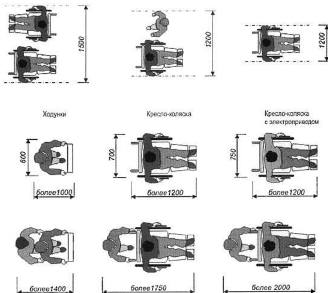
Рисунок В.12 - Параметры зон движения инвалидов
