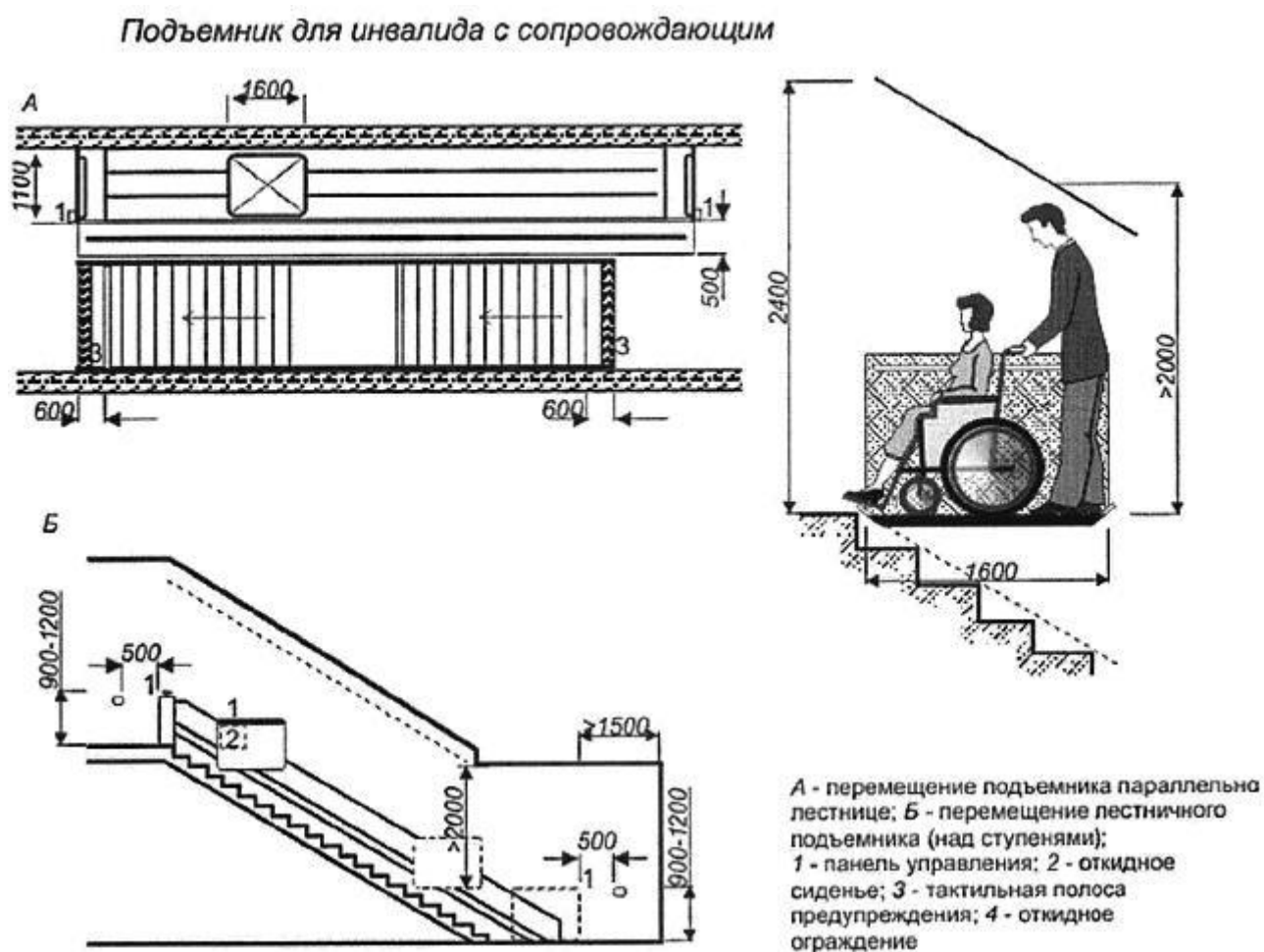
Рисунок В.31 - Параметры наклонных подъемников
