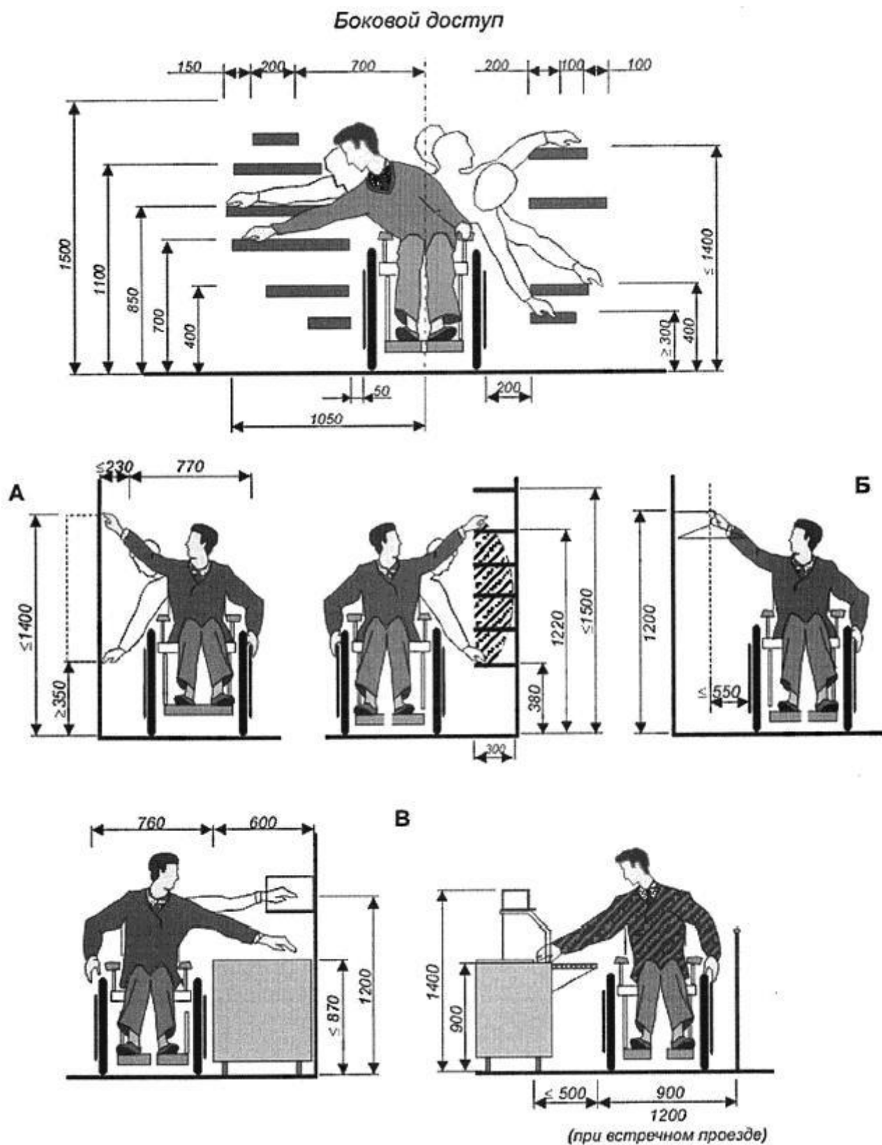
Рисунок Г.3 - Досягаемость в месте получения услуги
