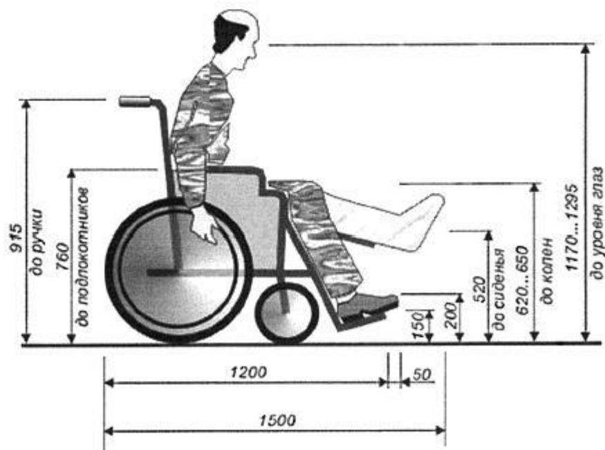
Рисунок В.1 - Габариты кресла-коляски
