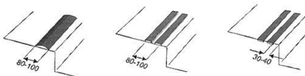
Параметры тактильных контрастных полос на ступенях
