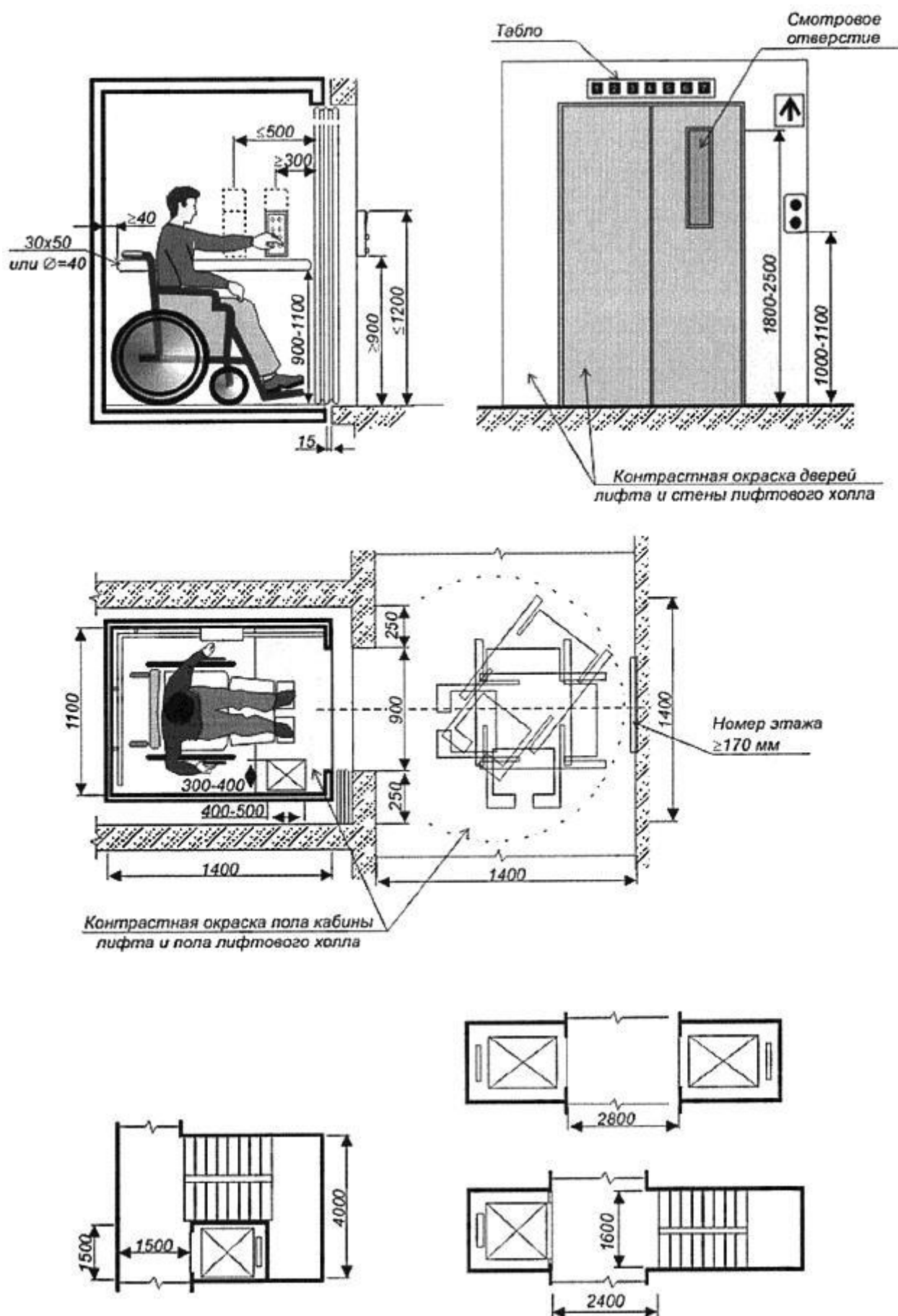
Рисунок В.30 - Оборудование лифтов
