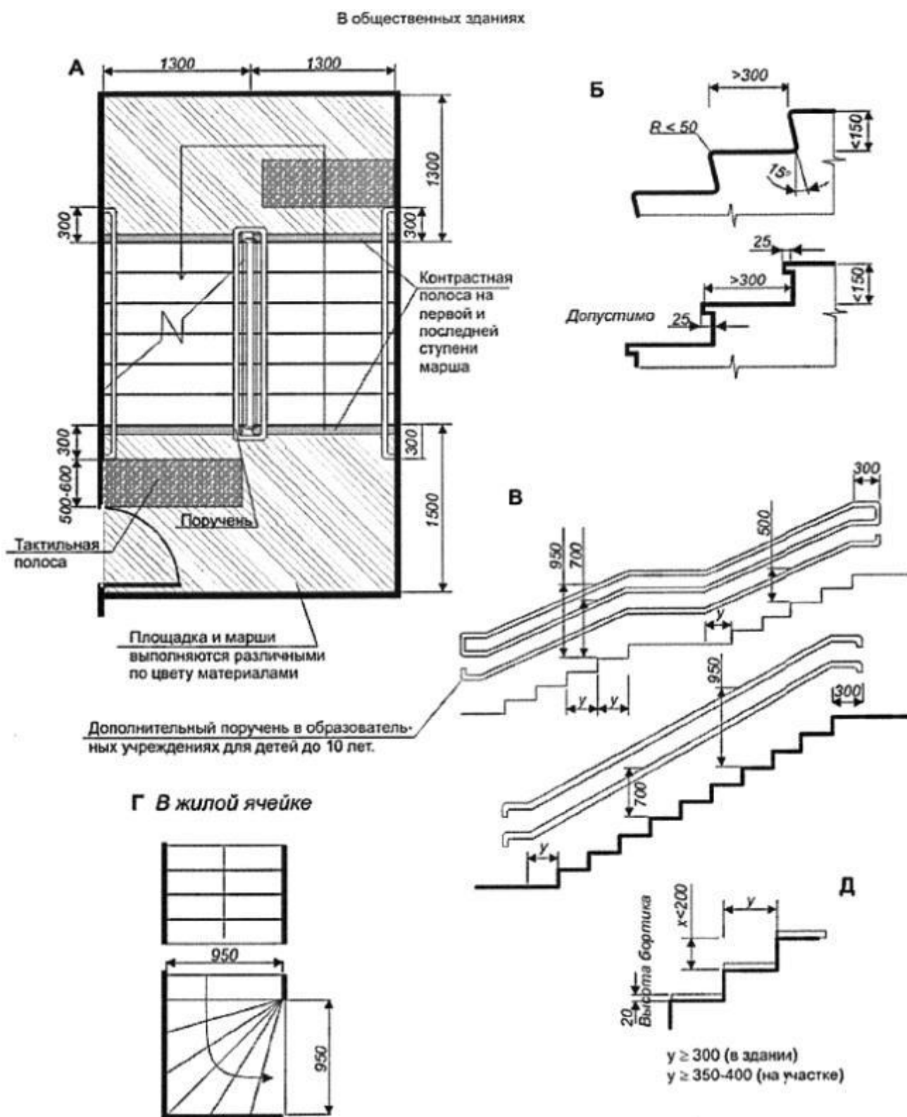
Рисунок В.23 - Лестницы в общественных зданиях и жилой ячейке
