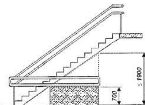
Предохранительная защита или поручни в зоне опасности
