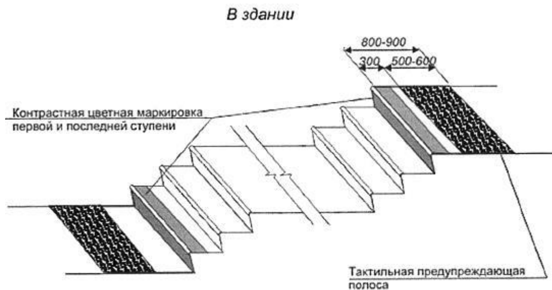
Рисунок В.22 - Предупреждающие контрастные и тактильные полосы
