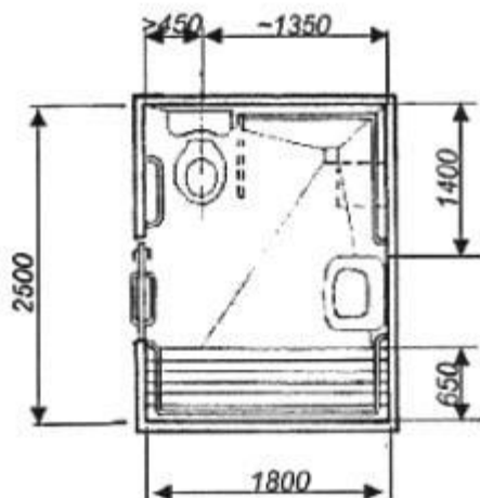
Непроходная кабина
