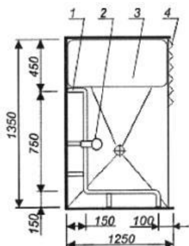
Рисунок Г.11 - Габариты душевых кабин
