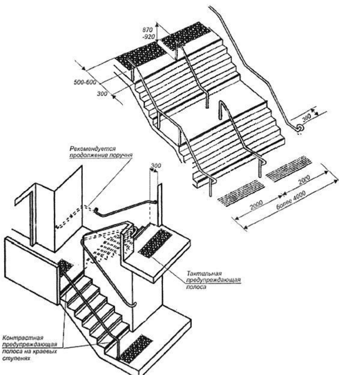
Предохранительная защита или поручни в зоне опасности
