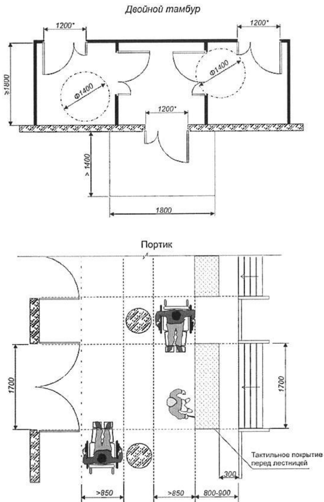
Рисунок В.21 - Площадки перед тамбуром и портиком
