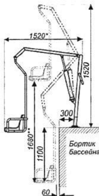
Рисунок Г.10 - Примеры конструкций подъемников для пересадки в ванну и бассейн
