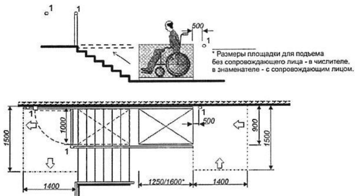
Подъемник для самостоятельного перемещения инвалида
