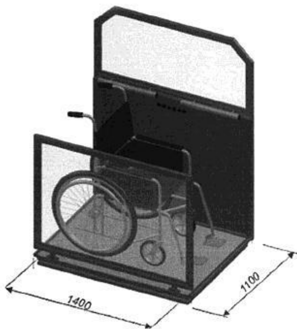
Рисунок В.33 - Параметры вертикальных подъемников
