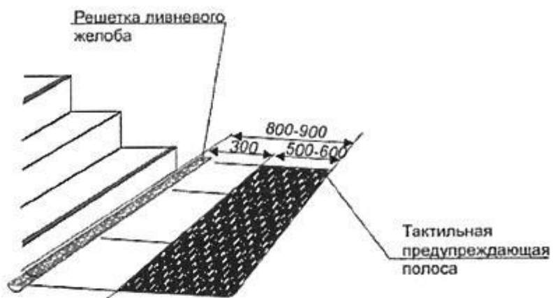
Параметры тактильных контрастных полос на ступенях
