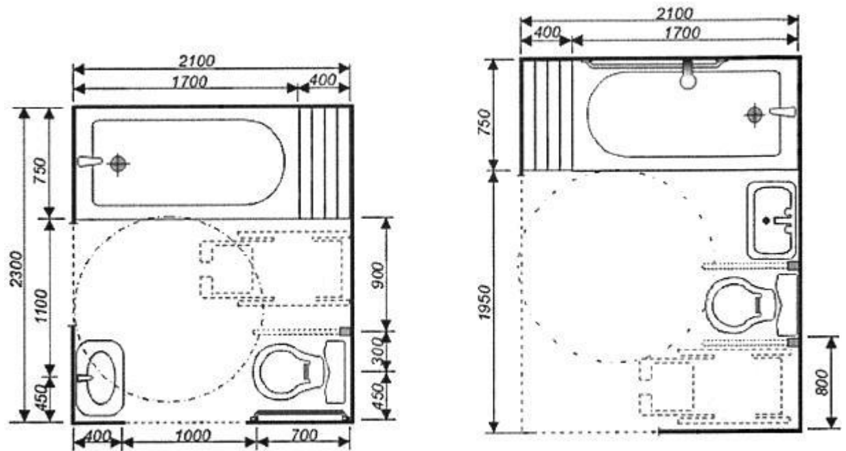
Рисунок Г.12 - Примеры оборудования совмещенного санитарного узла
