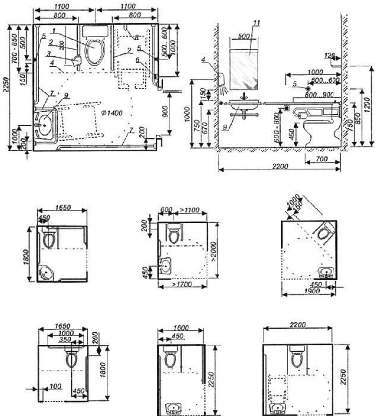
Рисунок Г.7 - Примеры оборудования кабин общественных уборных
