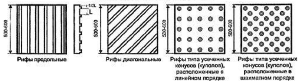
Типы рифления тактильно-контрастных указателей для технологии хоподного пластика
