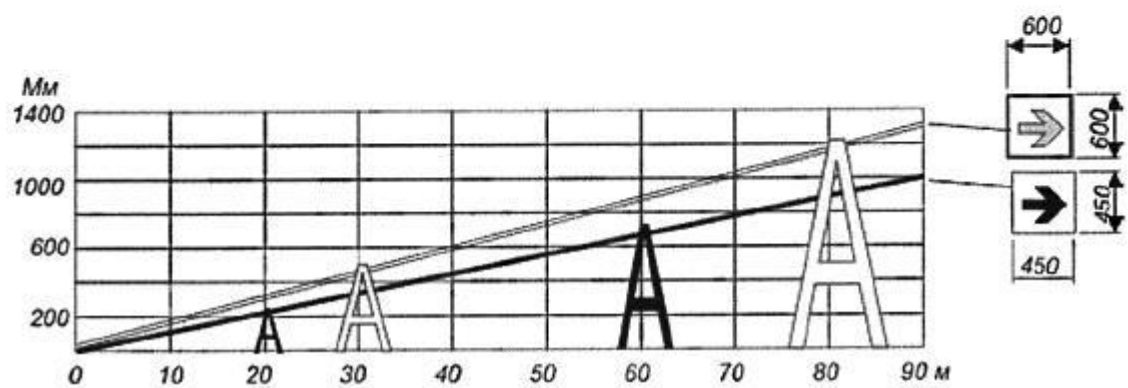
Зависимость размеров знака от контраста надписи
