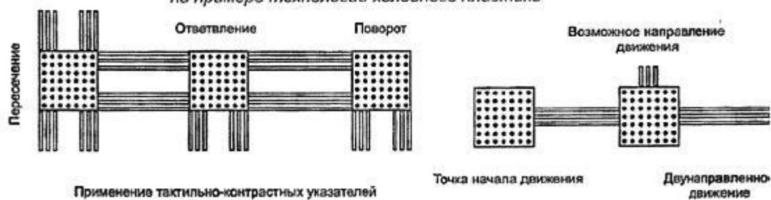
Применение тактильно-контрастных указателей на примере технологии холодного пластика
